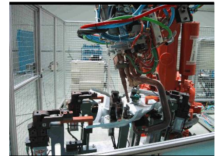
Robot con equipo de soldadura
