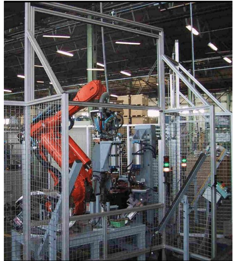
Robot de manipulación para cargar piezas unitarias en una cabina de soldadura
